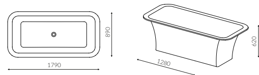
TYTAN WANNA / BATHTUB
