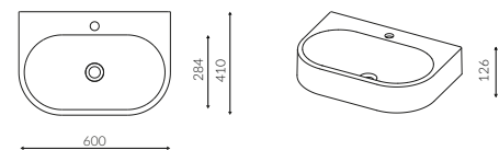
PIA 600 UMYWALKA / WASHBASIN
