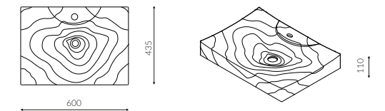
ROSA UMYWALKA / WASHBASIN
