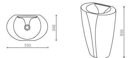
SELIA UMYWALKA STOJĄCA / STANDING WASHBASIN
