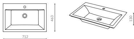
TEODOR UMYWALKA / WASHBASIN
