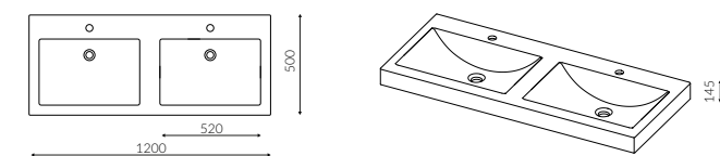
MOIRA BIS 120 DUET
