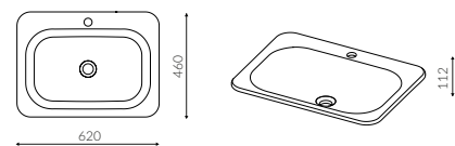
TYTAN UMYWALKA / WASHBASIN
