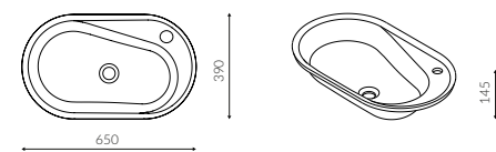
ALTA UMYWALKA / WASHBASIN
