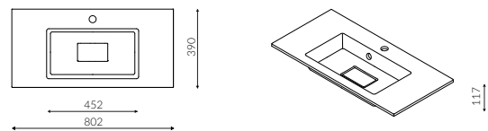
LIRA 900 LEWA/ PRAWA / LEFT/ RIGHT
