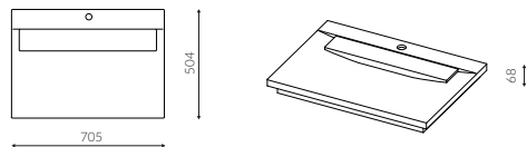
TATOO BIAŁA PŁYTKA / WHITE PLATE
