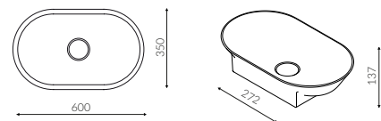
LIVA 600 UMYWALKA / WASHBASIN
