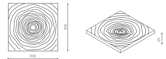
ROSA 90 BRODZIK KWADRATOWY / SQUARE SHOWER TRAY
