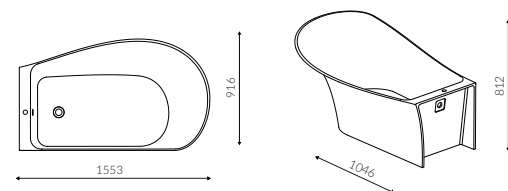
MISA LEWA / LEFT WANNA NAROŻNA / CORNER
