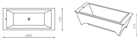
TEODOR WANNA Z ZABUDOWĄ / BATHTUB WITH ENCLOSURE
