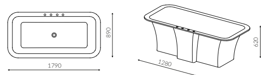
TYTAN WANNA Z ZABUDOWĄ / BATHTUB WITH ENCLOSURE
