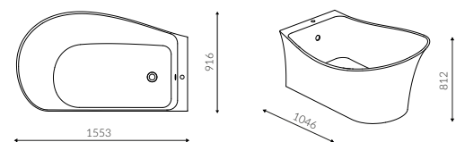
MISA LEWA / LEFT WANNA NAROŻNA / CORNER
