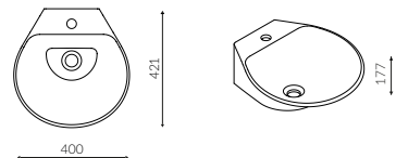
MISA PRAWA / RIGHT WANNA NAROŻNA / CORNER BATHTUB
