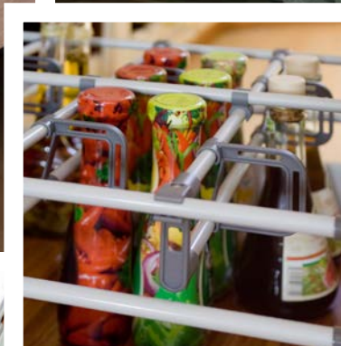
FDS-DF A duplafalú fém fiókoldal FDS-DF B duplafalú fém fiókoldal oldalmagasítóval
