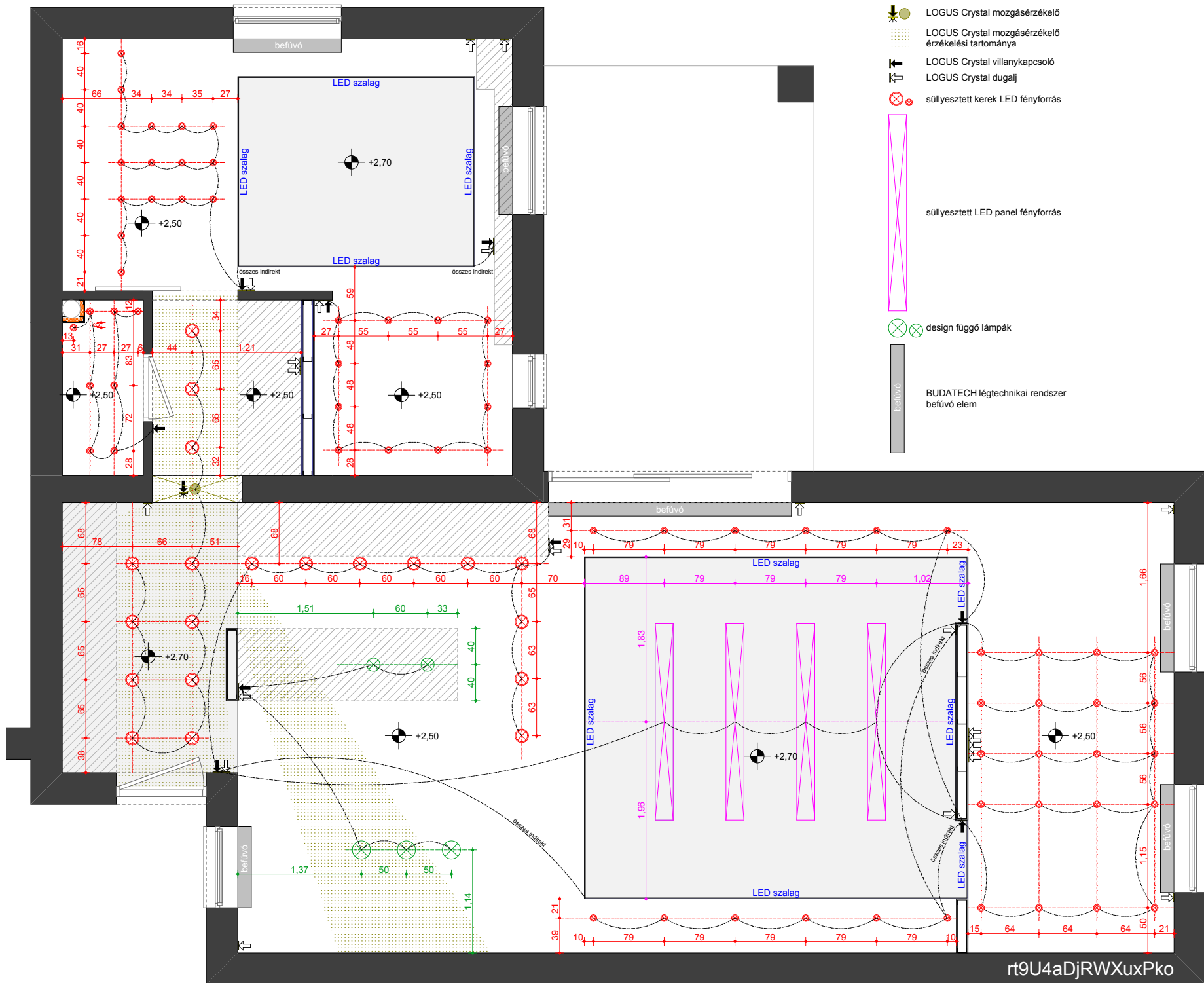
KAPCSOLÁSI ÉS VILÁGÍTÁSI RAJZ M 1 : 50
