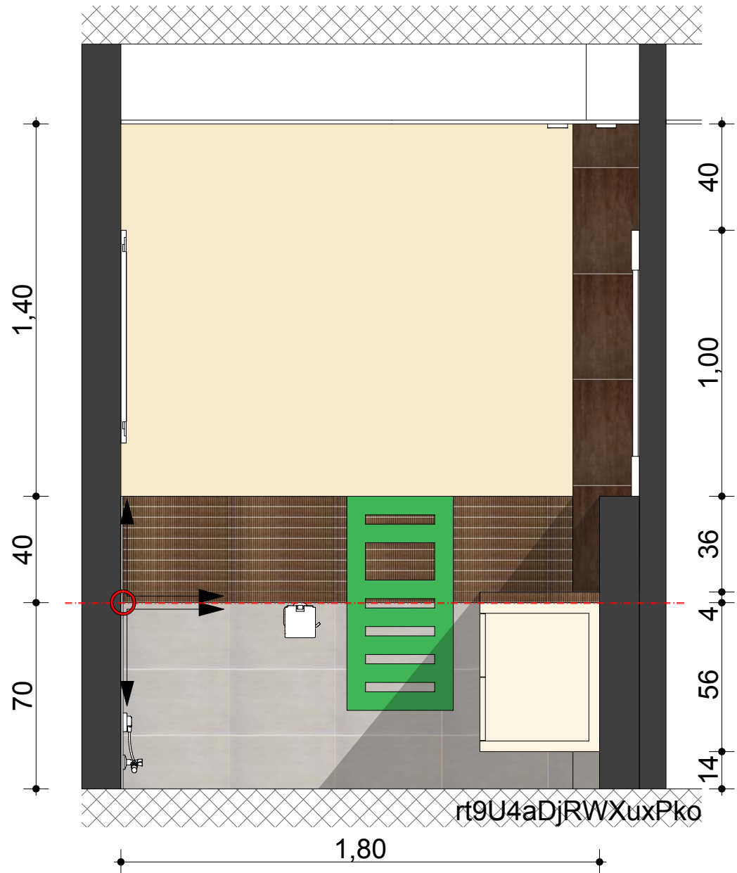
WC BURKOLÁSI TERV 1 M 1 : 20
