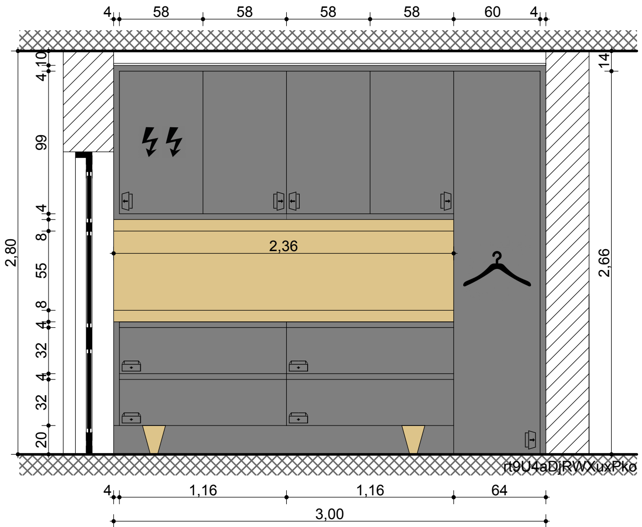
ELŐSZOBA BÚTOR TERV M 1 : 25
