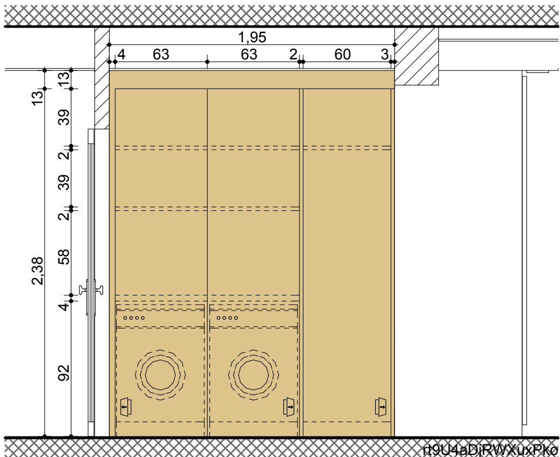
HÁZTARTÁSI BÚTOR TERV M 1 : 25
