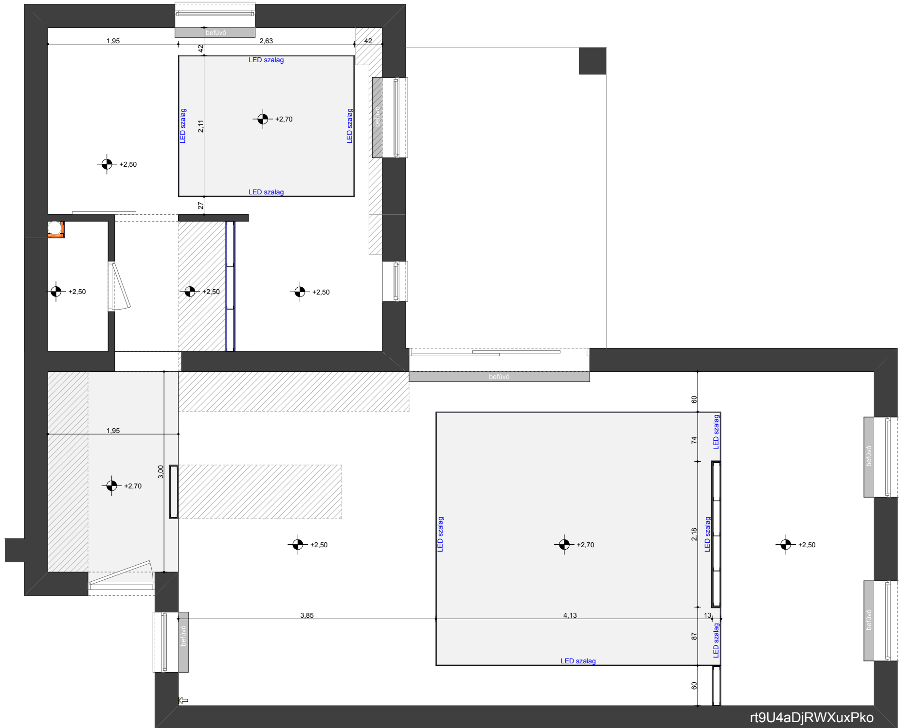
ÁLMENYEZETI TERV M 1 : 50
