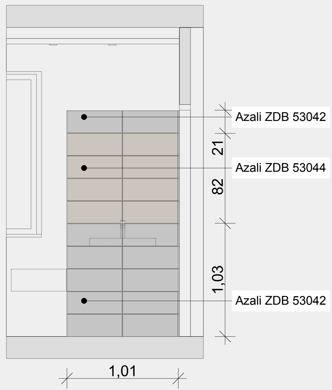
F1 JELŰ FALNÉZET
