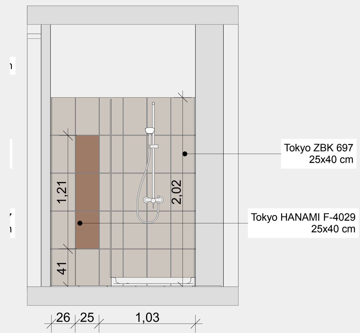
Z3 JELŰ FALNÉZET
