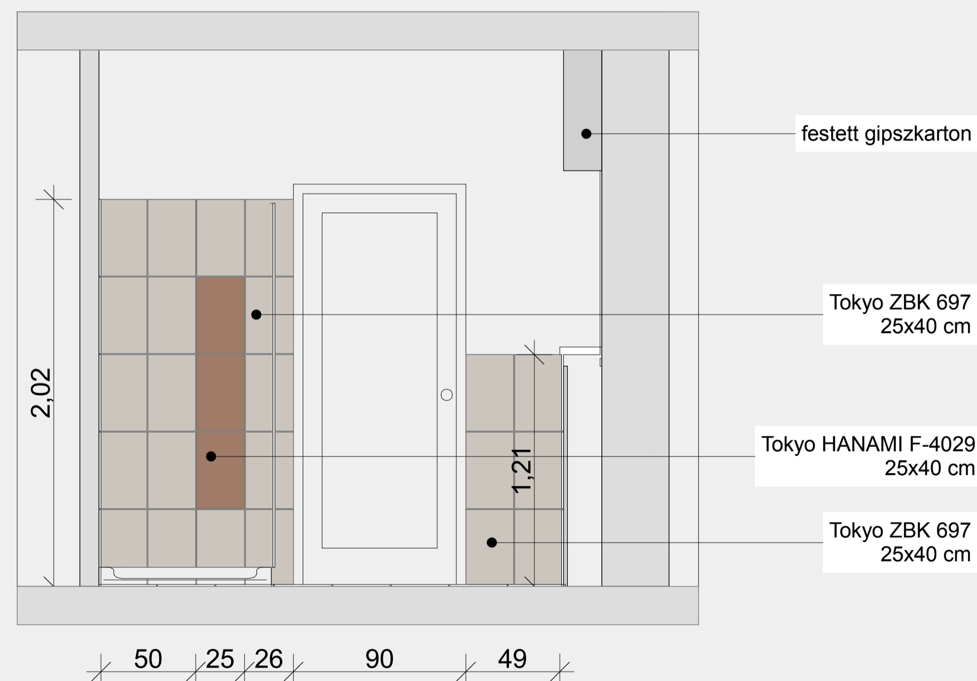
Z4 JELŰ FALNÉZET
