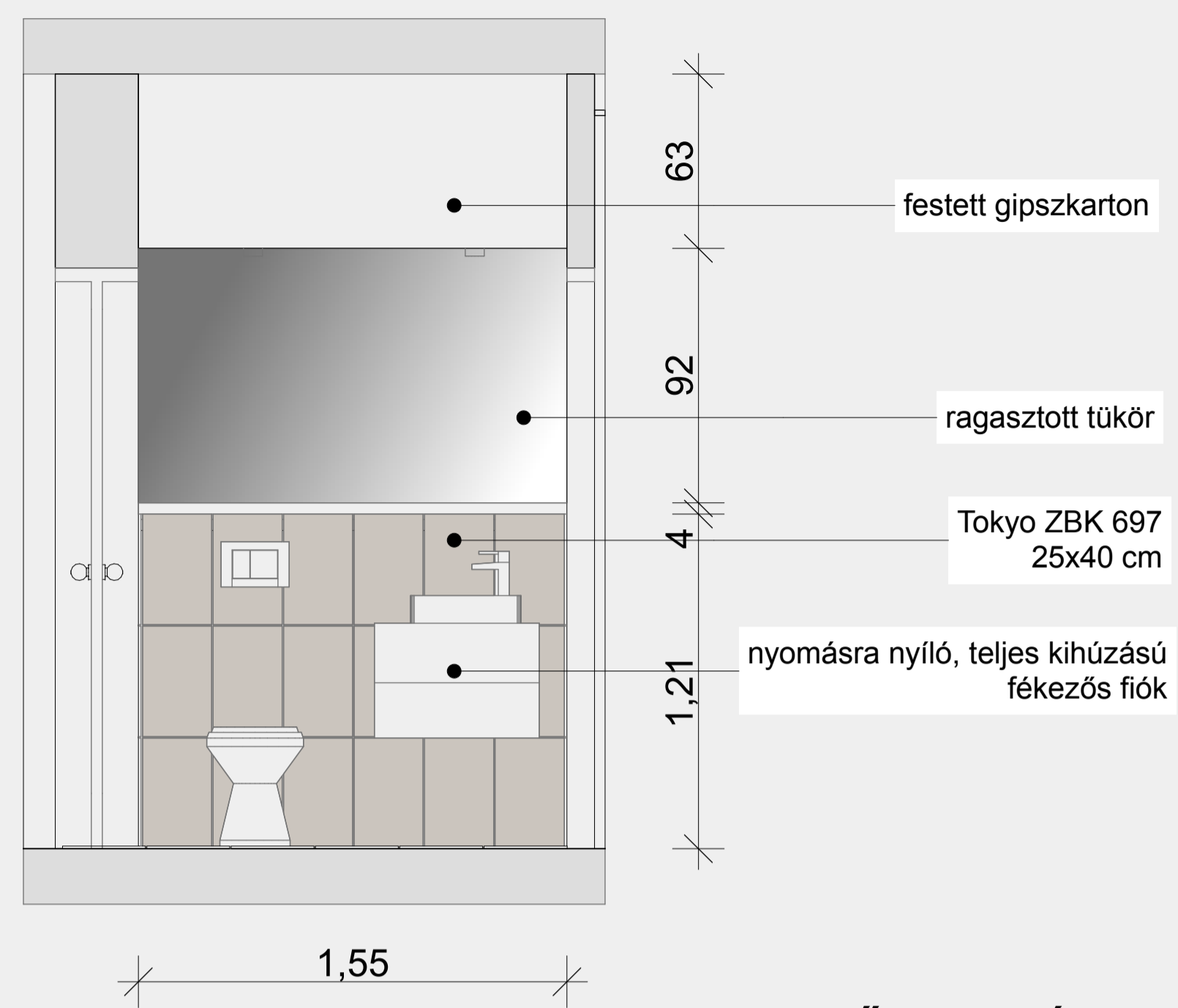
Z1 JELŰ FALNÉZET
