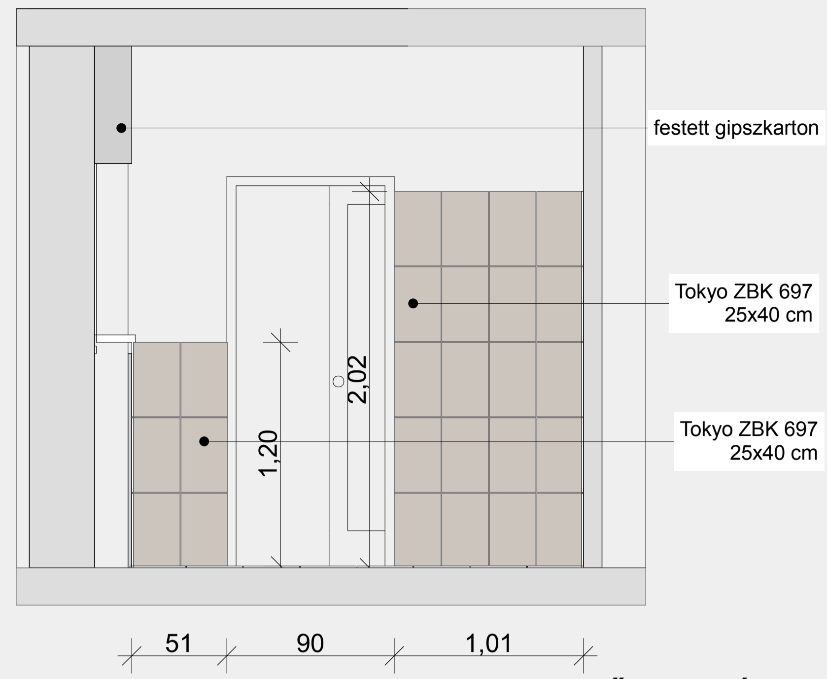
Z2 JELŰ FALNÉZET
