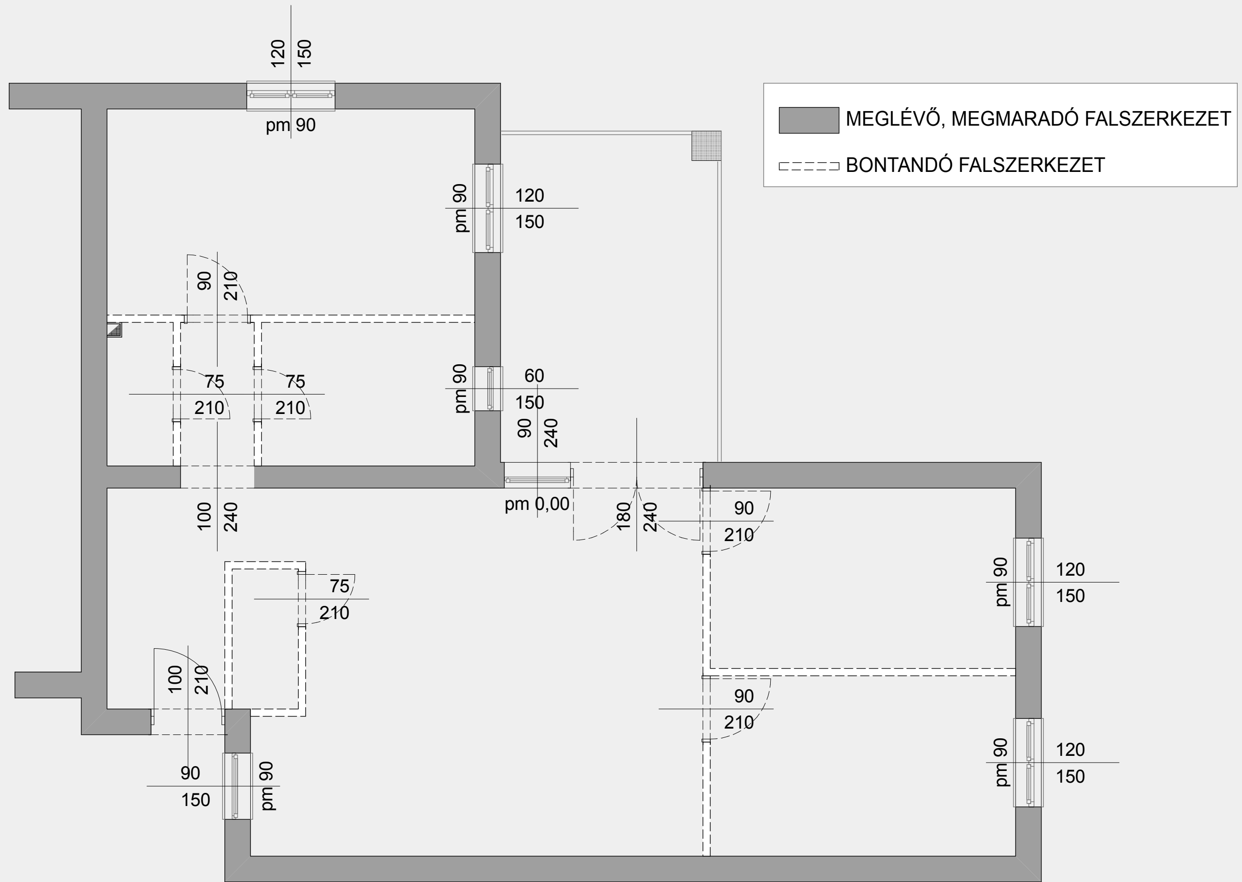
BONTÁSI TERV M 1:50
