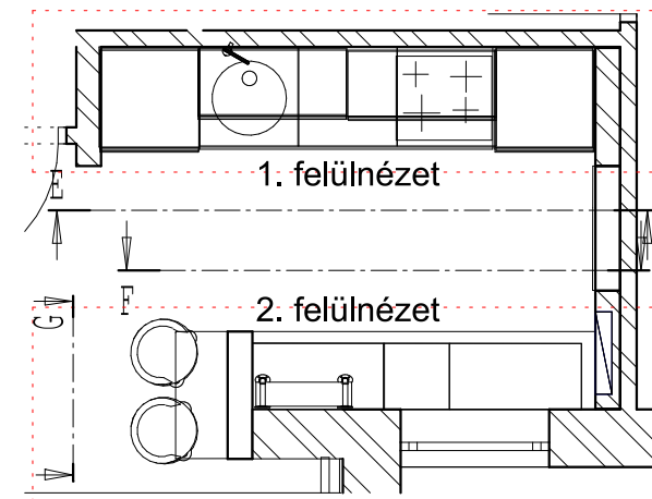
Alaprajz részlet - Konyha
