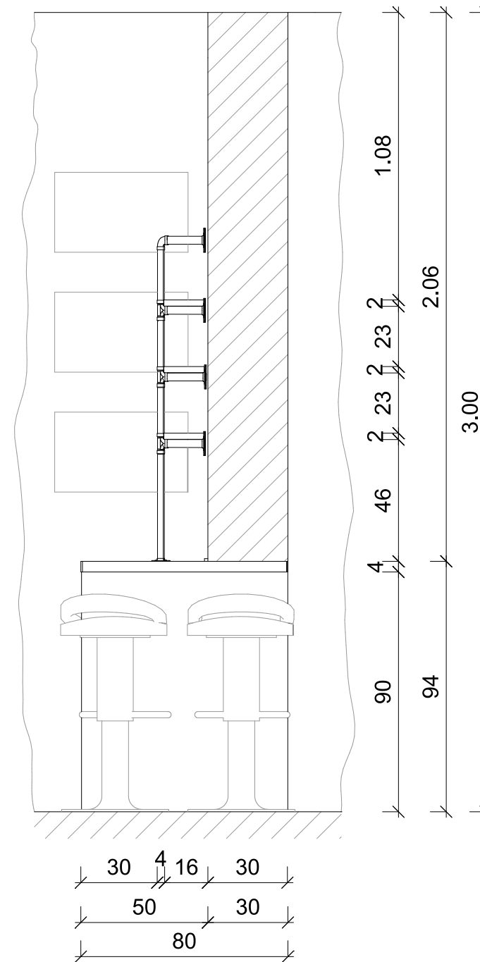
G - G Metszet oldalnézet
