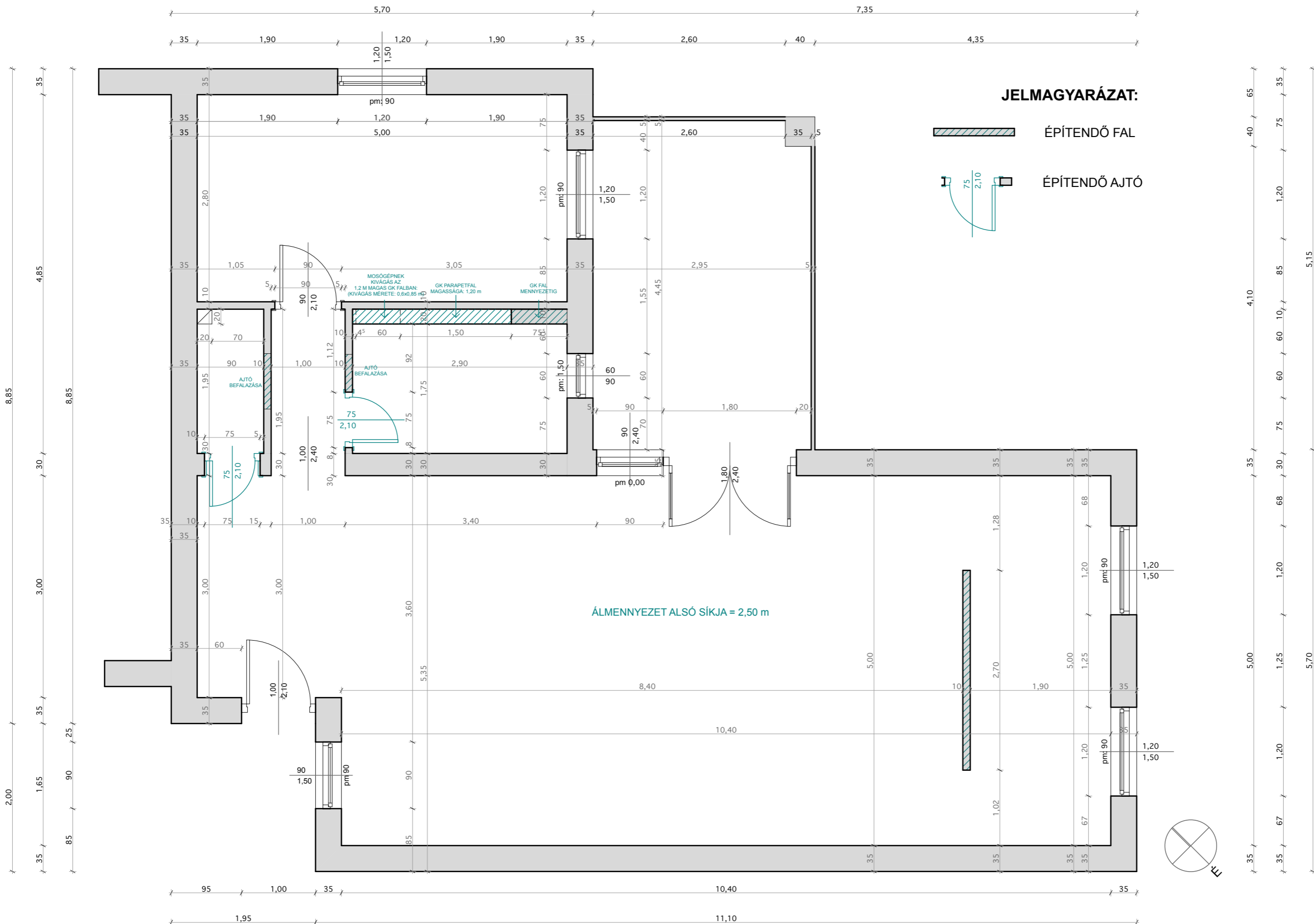
ÉPÍTÉSI ALAPRAJZ
