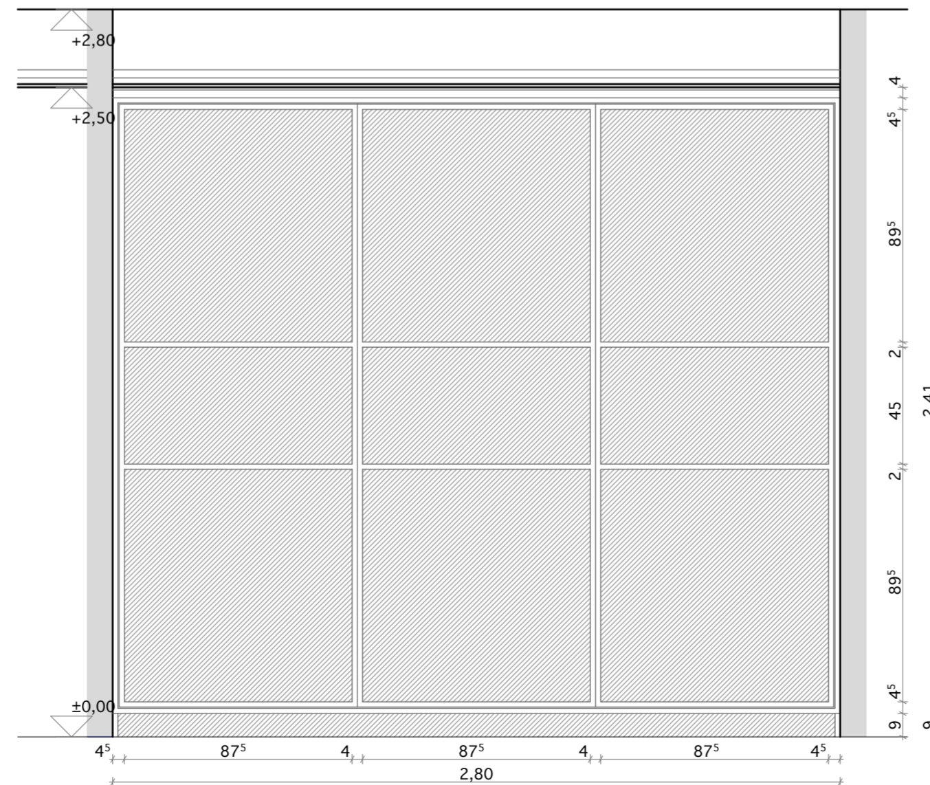
GARDRÓBSZEKRÉNY HÁLÓSZOBÁBAN: M: 1:20
