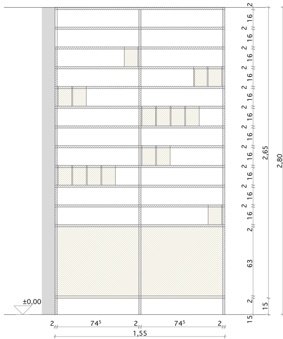
VIRÁGTARTÓ ÁLLVÁNY AZ ERKÉLYEN: M: 1:20
