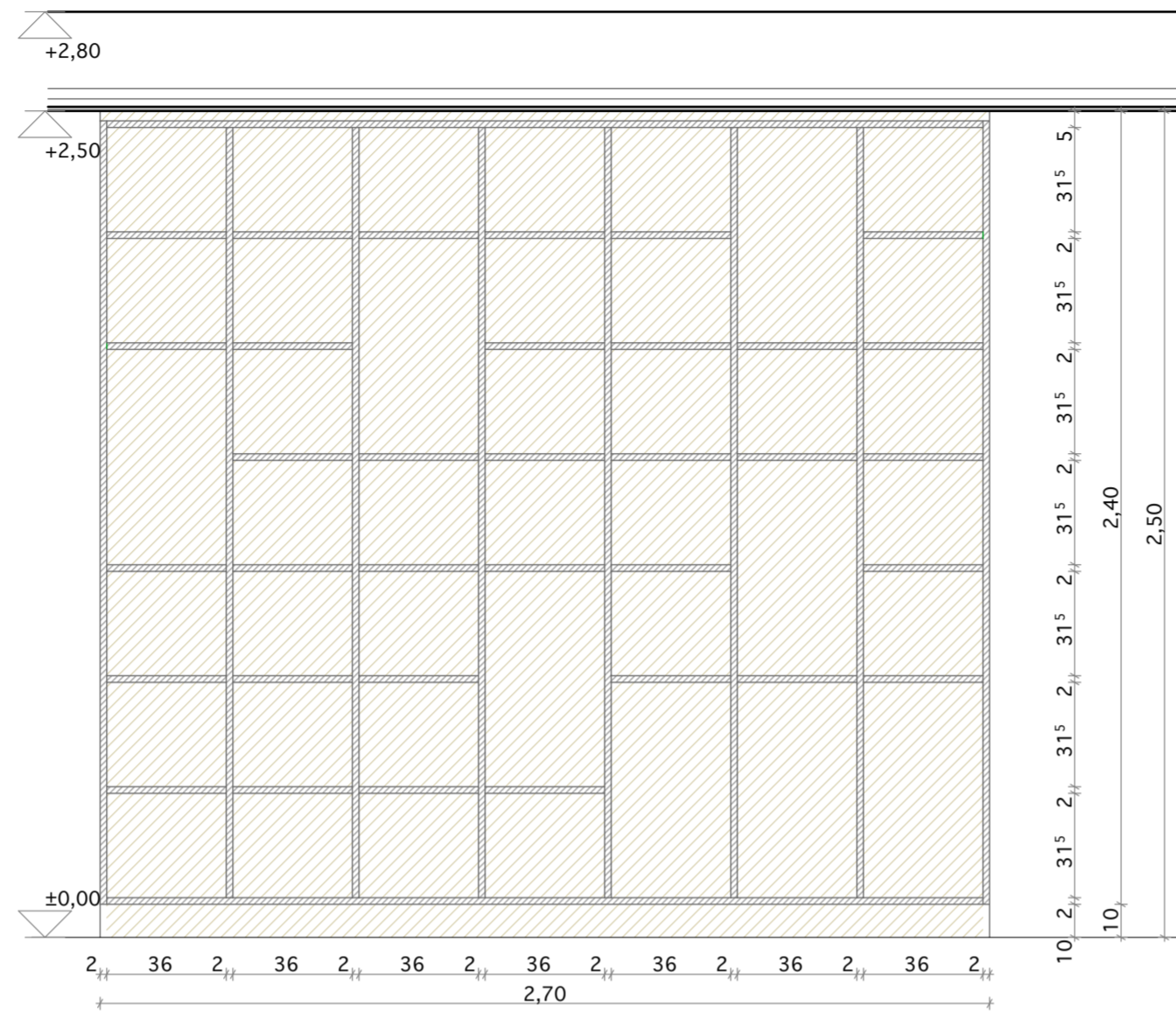
SZEKRÉNY A DOLGOZÓSAROKBAN: M: 1:20
