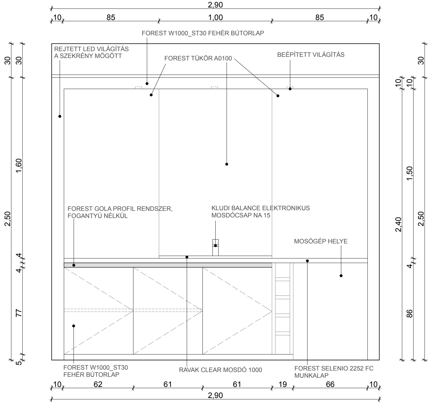
FÜRDŐ EGYEDI BÚTOR FALNÉZET B
