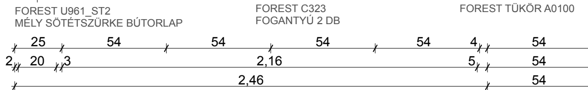
ELŐTÉR EGYEDI BÚTOR FALNÉZET
