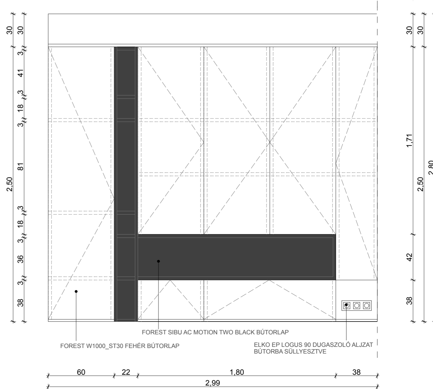
NAPPALI EGYEDI BÚTOR FALNÉZET B
