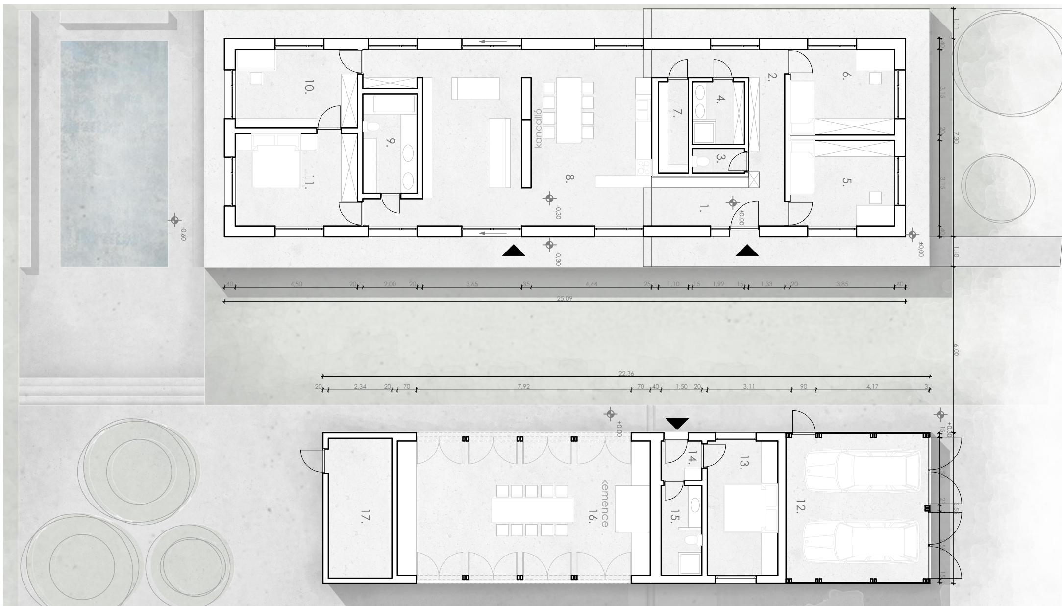
földszinti alaprajz
