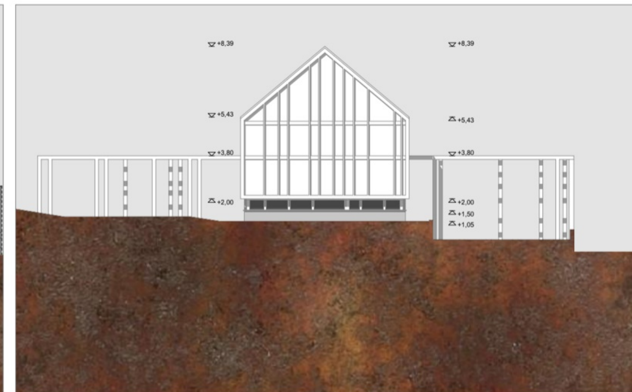
ÉSZAKI (UTCAI) HOMLOKZAT M = 1:100
