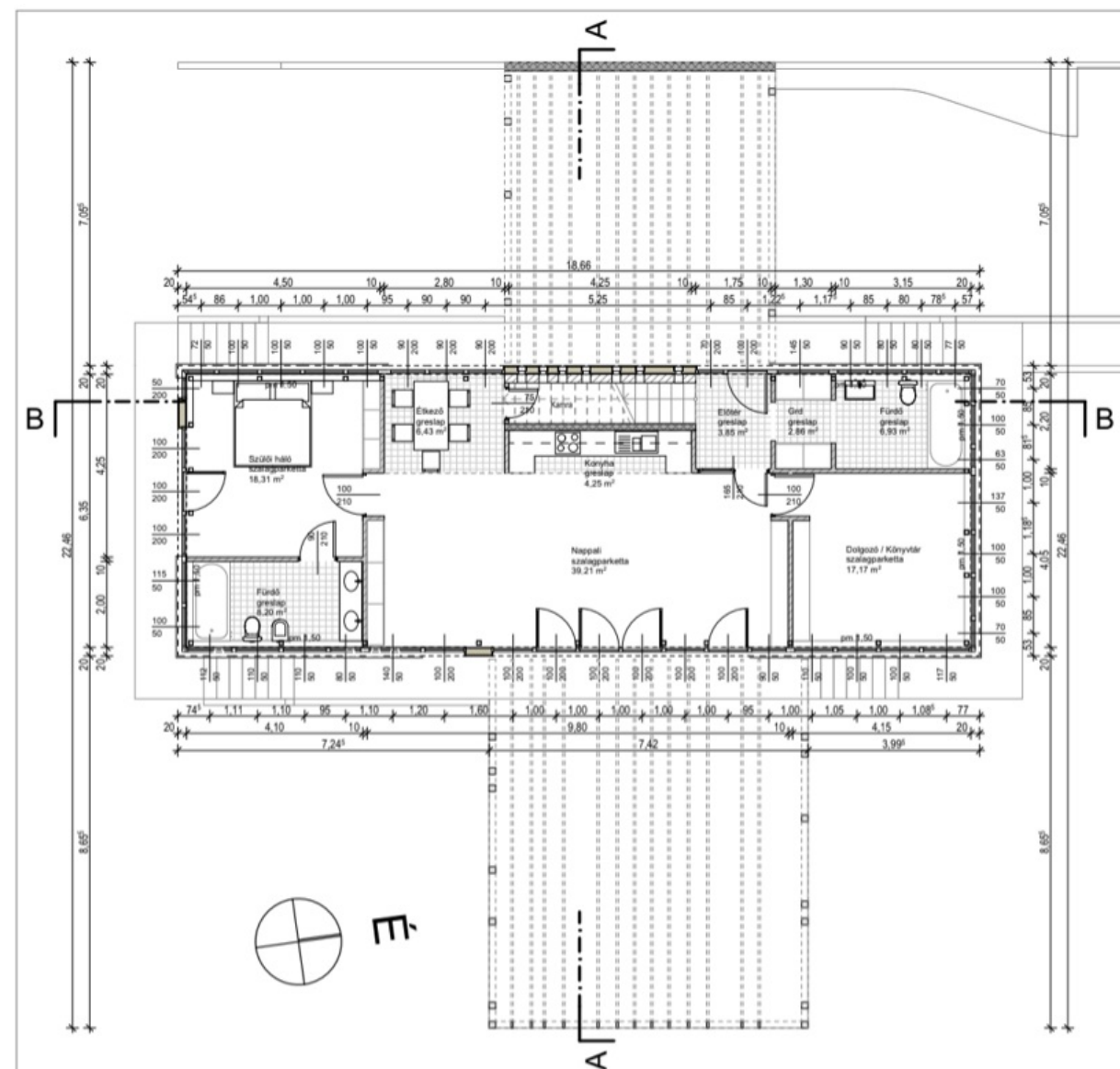
FÖLDSZINT ALAPRAJZA M = 1:100
