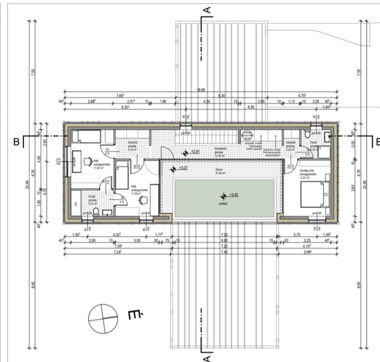
EMELET ALAPRAJZA M = 1:100
