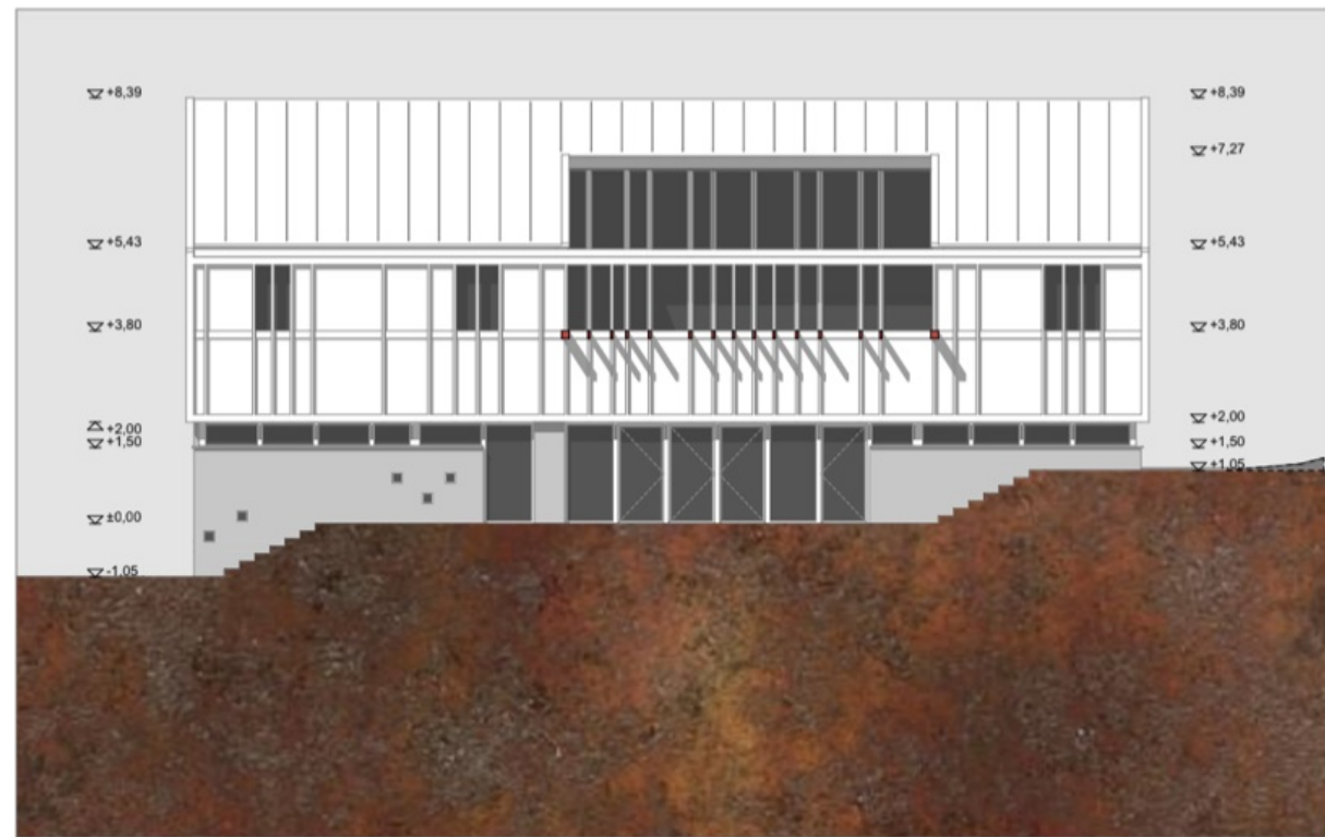
KELETI HOMLOKZAT M = 1:100
