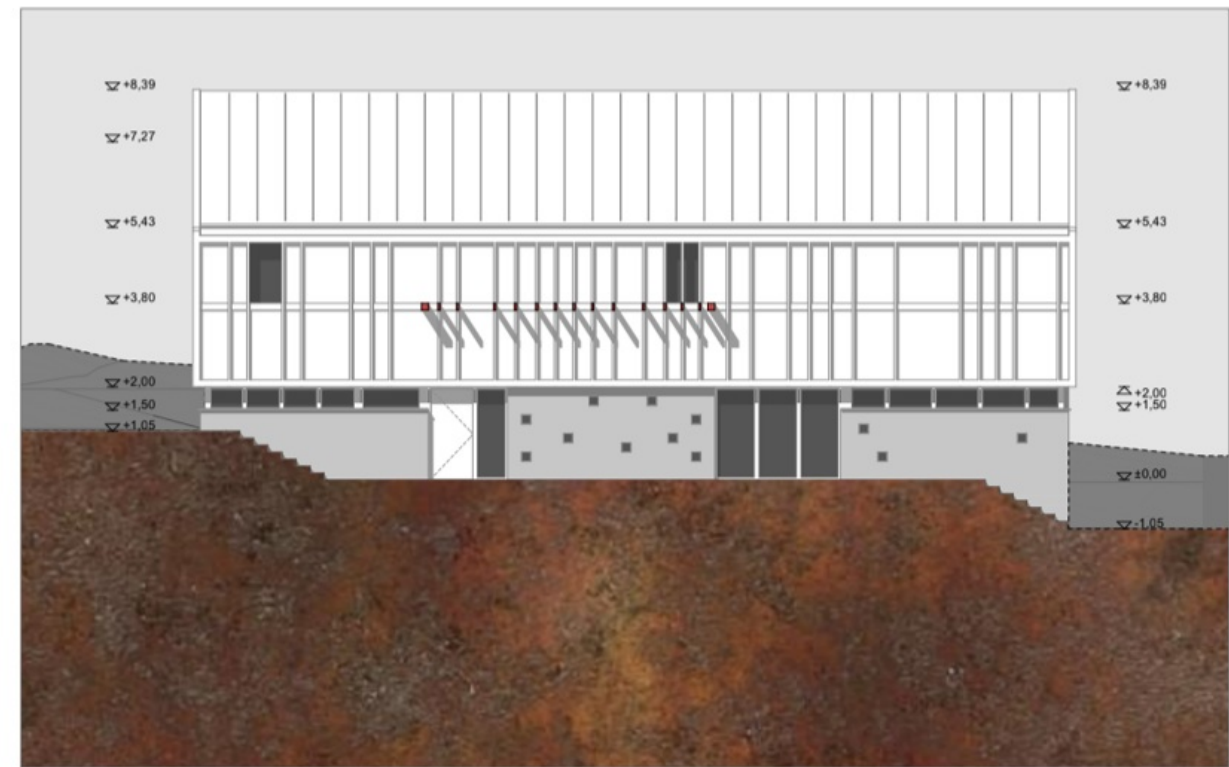
NYUGATI HOMLOKZAT M = 1:100
