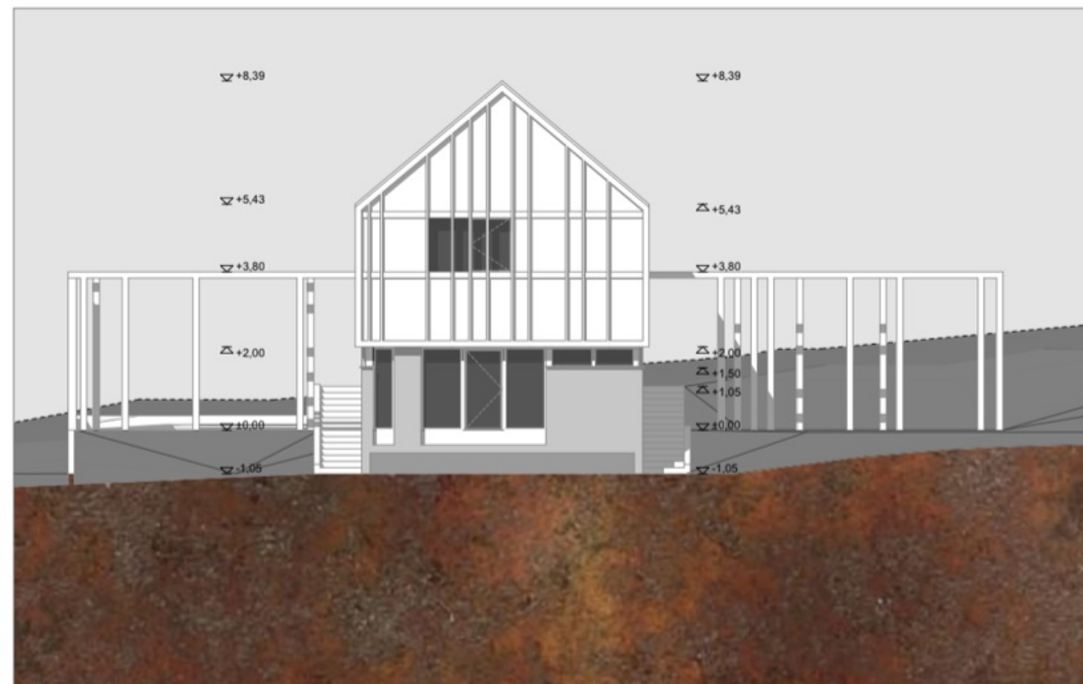
DÉLI HOMLOKZAT M = 1:100
