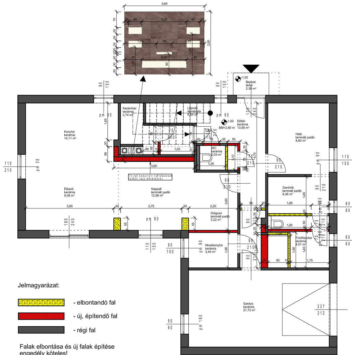
Építés - bontási terv méretezve - földszint (m=1:100)
