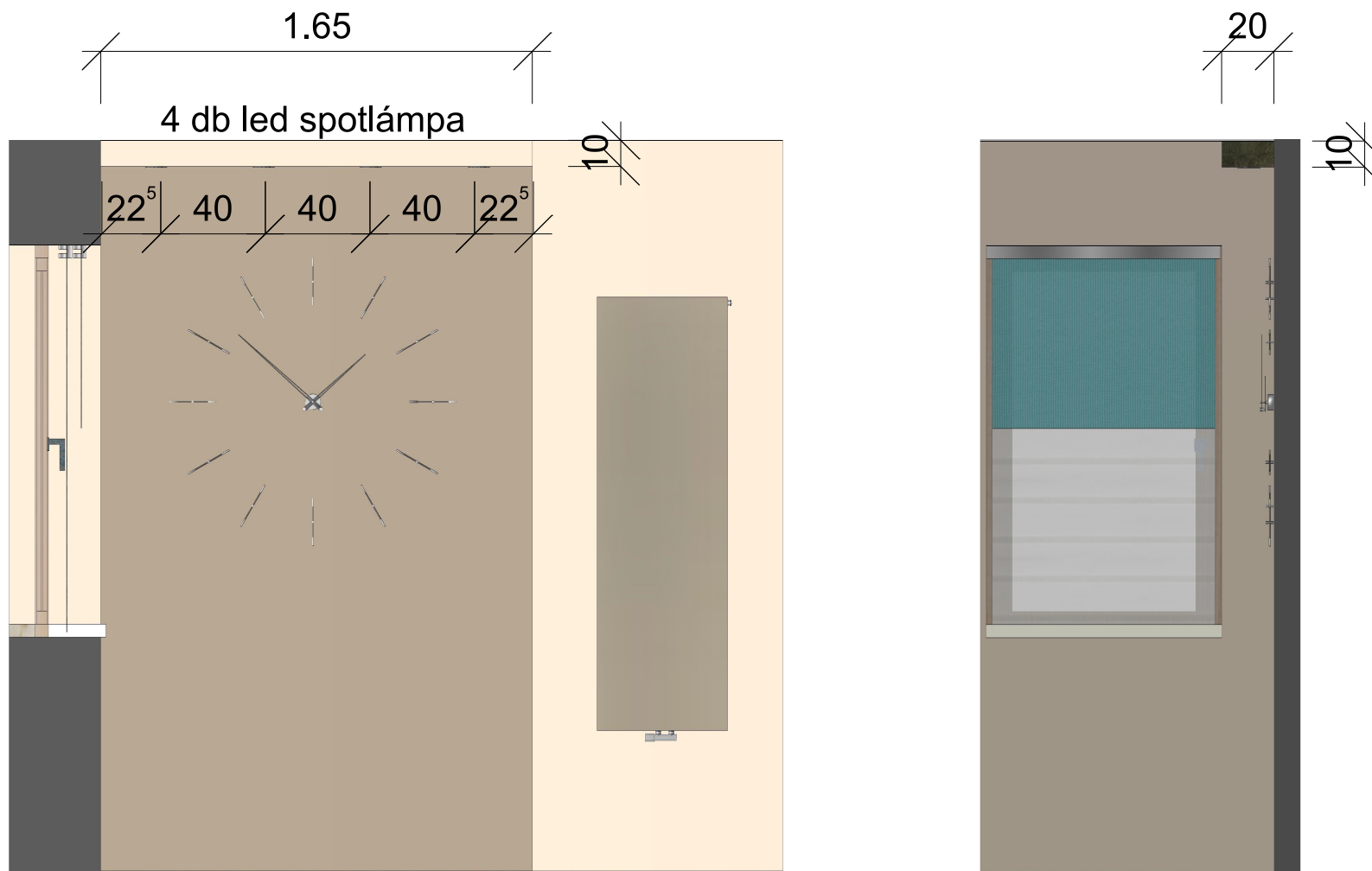
Álmennyezet Rigips gipszkartonból a konyha egyik falánál rejtett világításokkal
